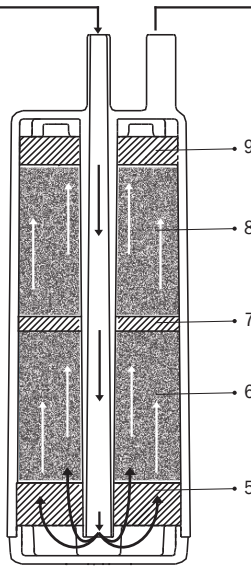
Filtro Cinco estágios
